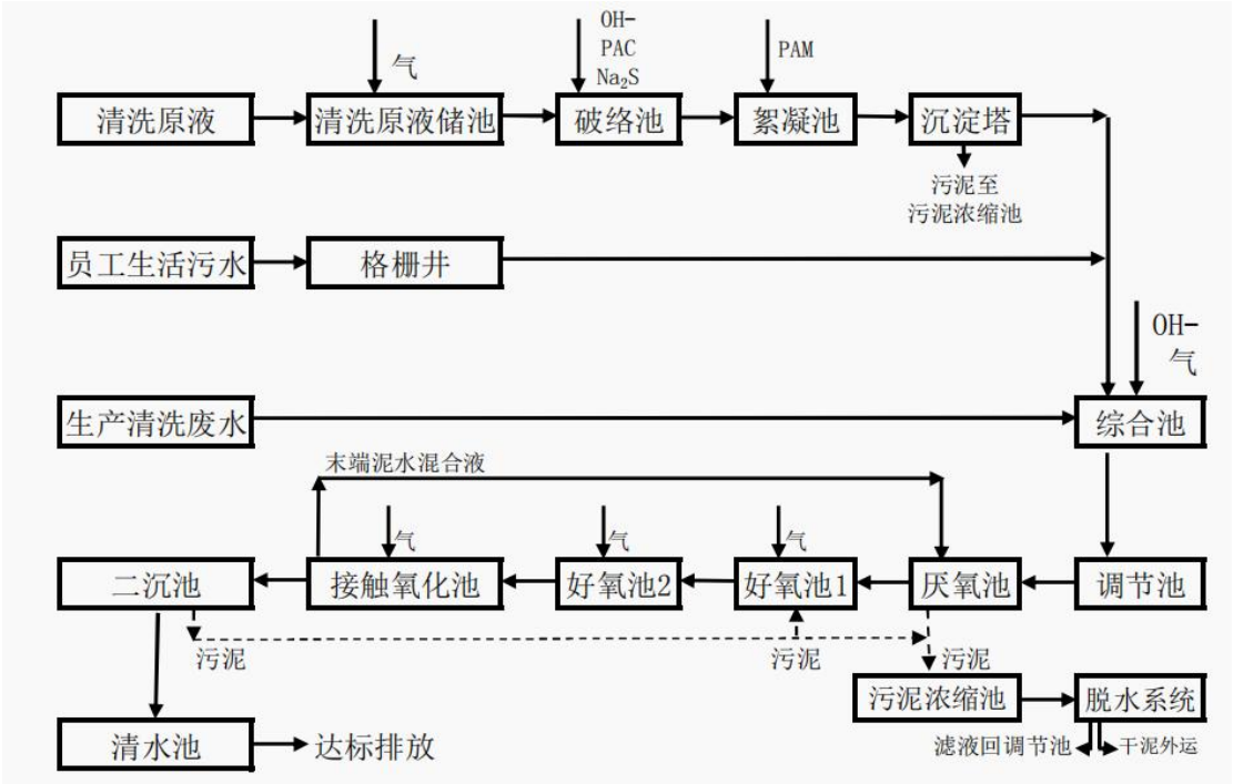
图 4.3-2 污水处理工艺流程图
